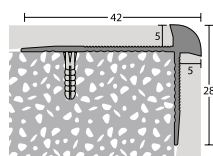
Terminal Degrau Stair nosing Perfilé nez-de-marche
